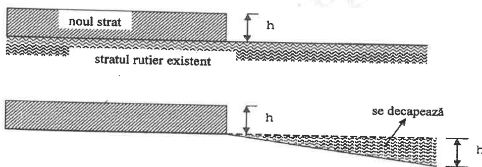
Fig. 1 Racordarea in profil longitudinal a stratului nou cu stratul existent
